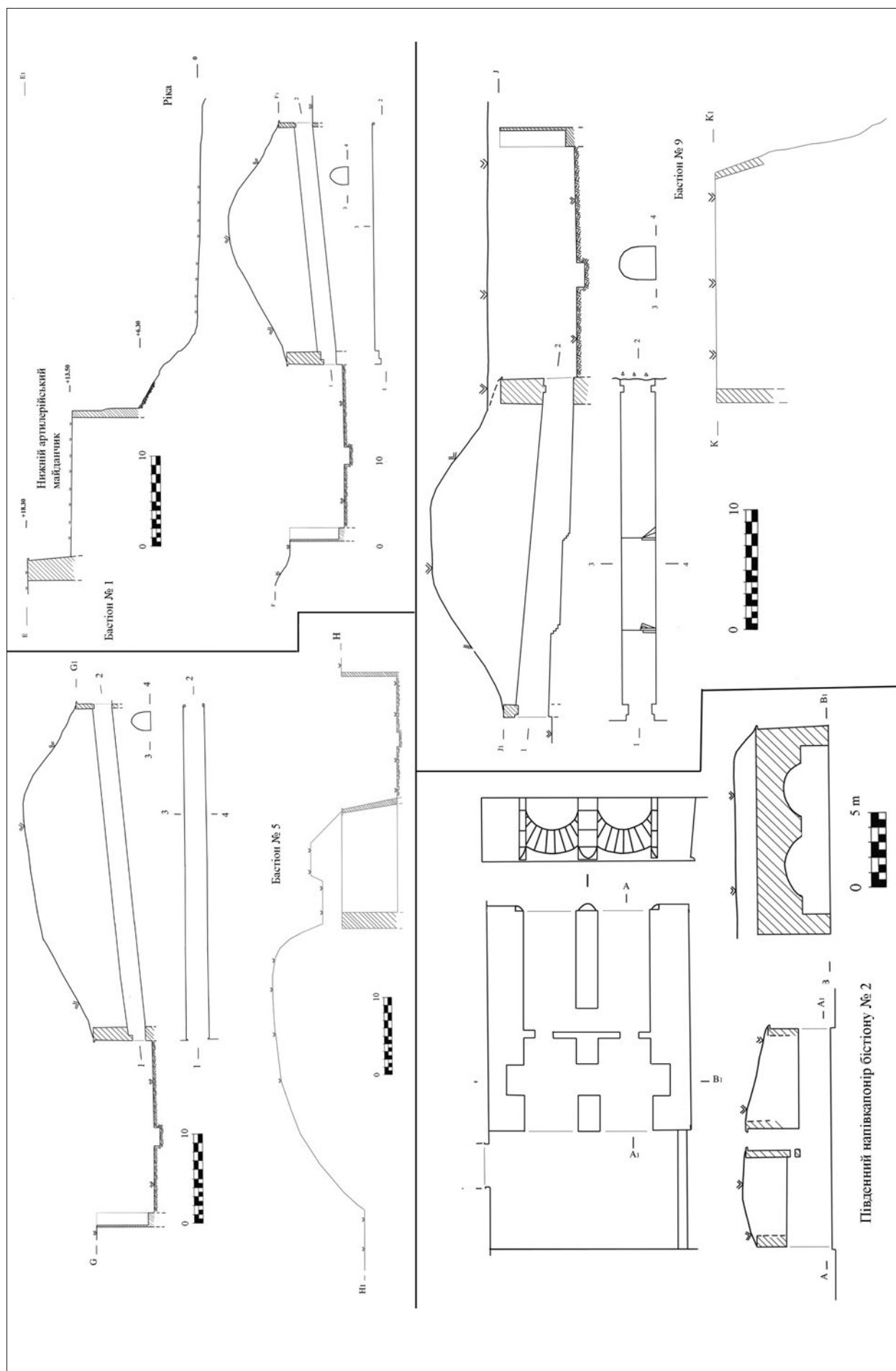
Рис. 69. Профілі валів Бендерської фортеці за обмірним планом фортеці.
