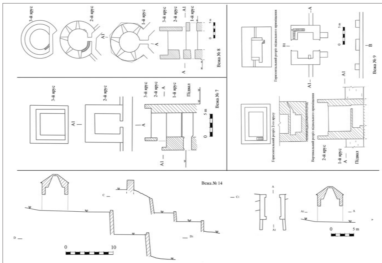
Рис. 60. Обмірні плани і розрізи веж № 7-9 цитаделі фортеці Бендери та вежі №14.
