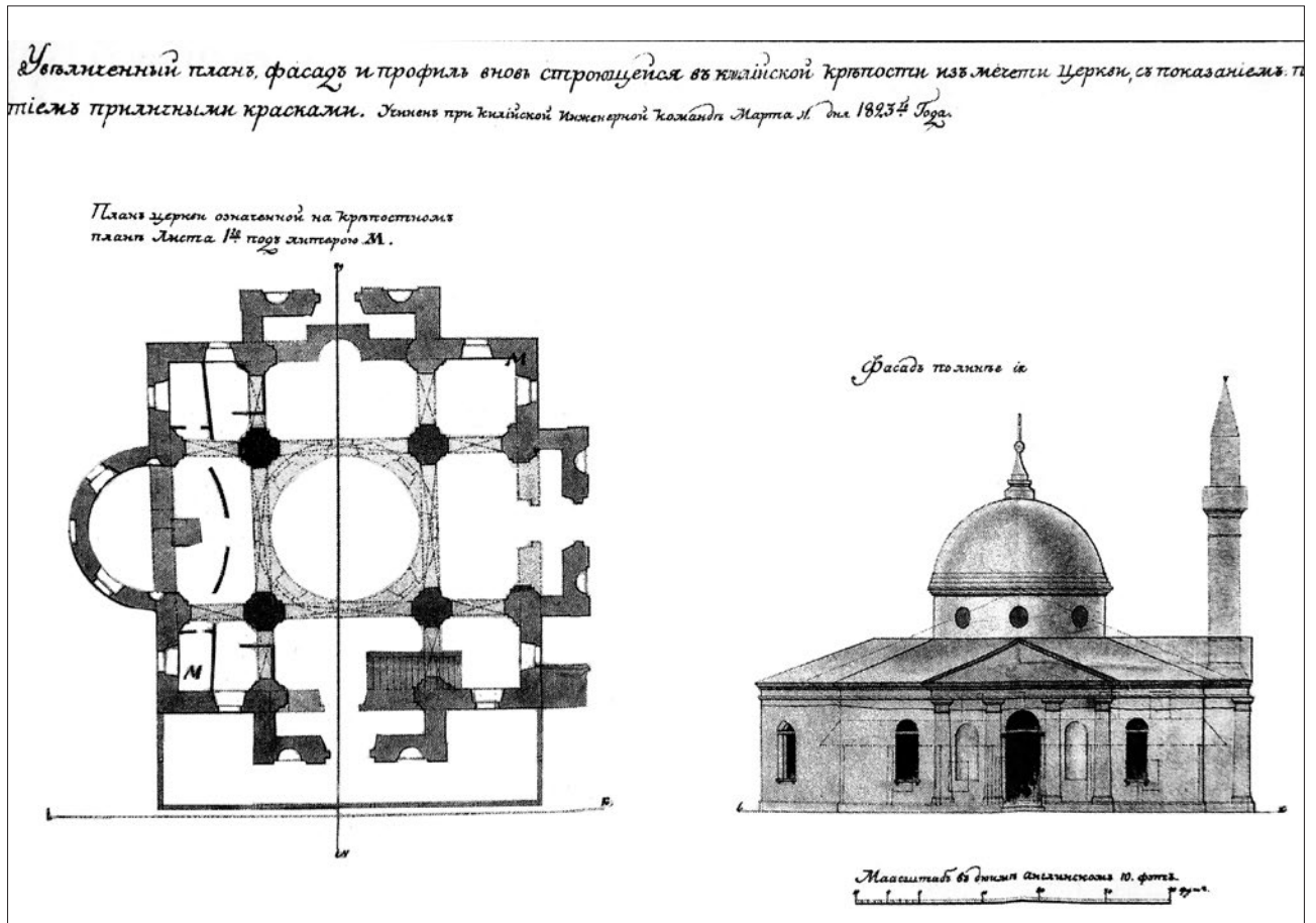
Рис. 158. Мечеть Баязида II у Кілії після перетворення на церкву (1823 р.). План і фасад (Şlaras 2016, р. 241).
