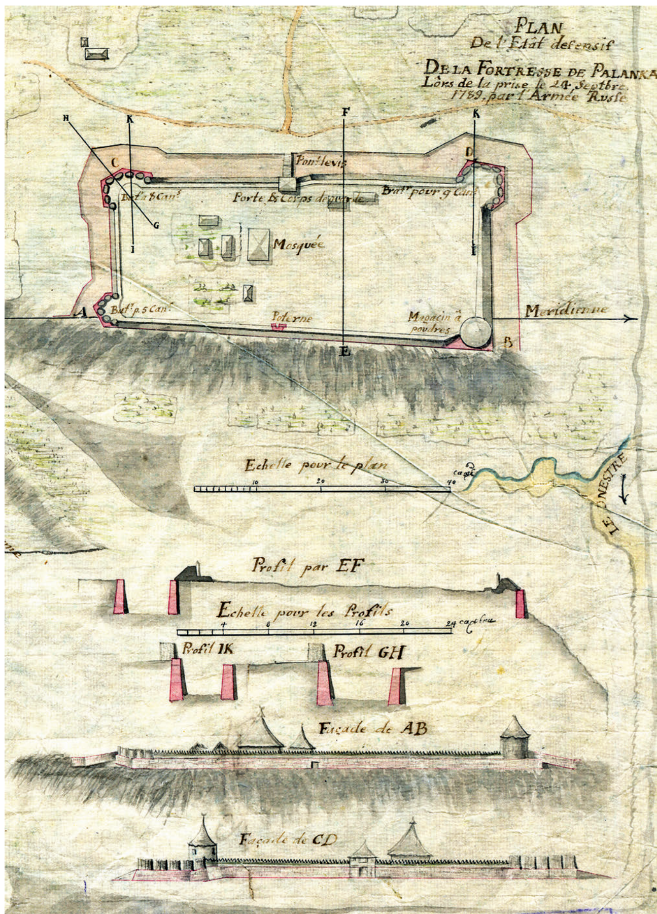
Рис. 26. Паланка. Креслення та розгортка фасаду фортеці. Фрагмент плану 1789 р.
