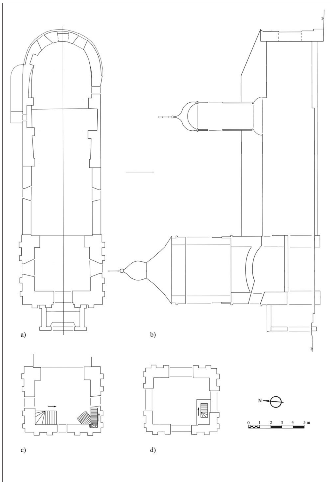
Рис. 149. Грецька церква Аккермана. Обмірний план.
