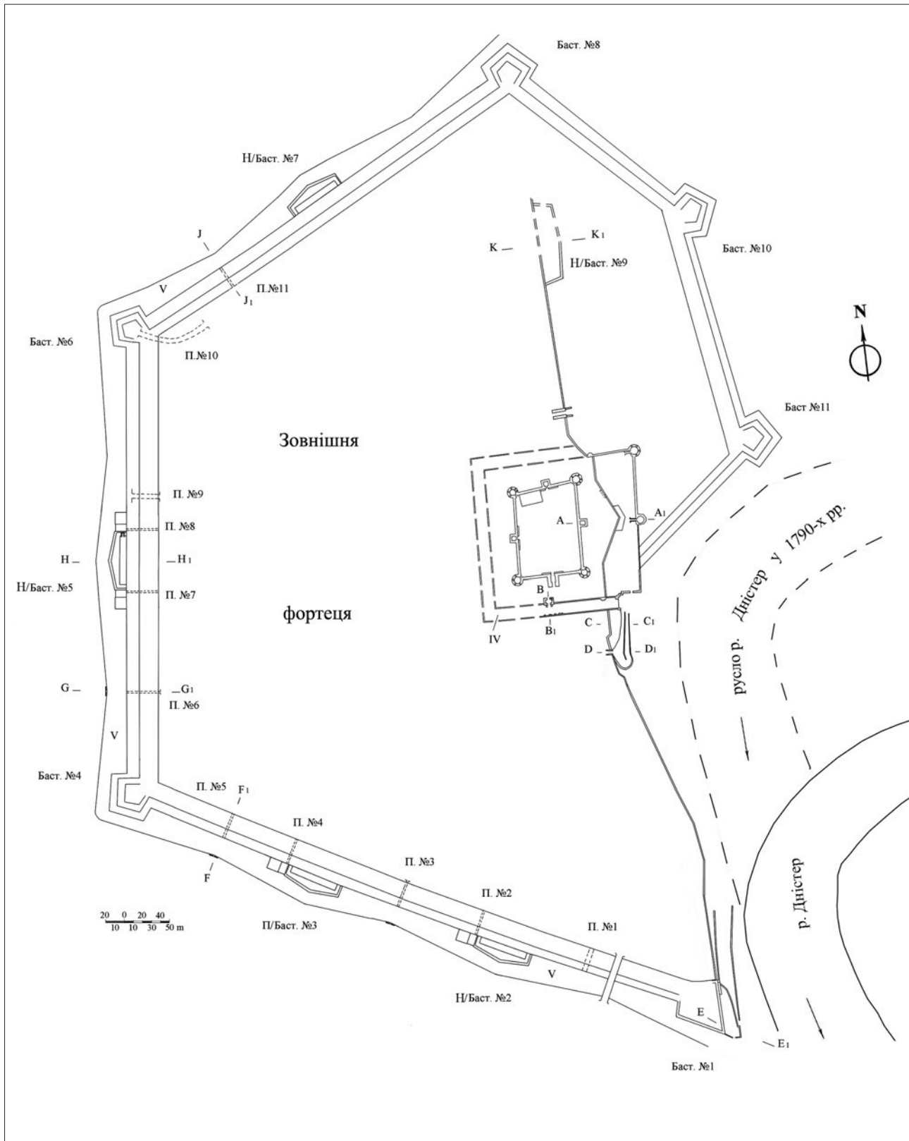
Рис. 68. Фортеця Бендери. Обмірний план оборонного комплексу (Красножон 2011а, с. 222).
