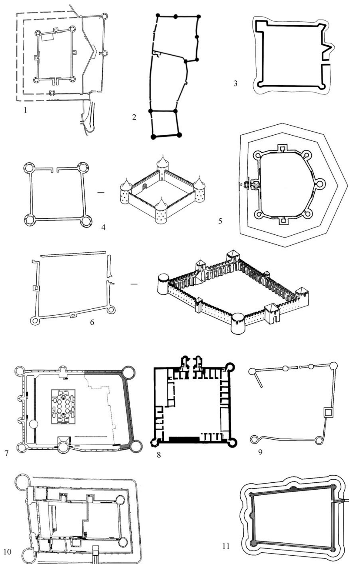
Рис. 46. Типологічні порівняння планів османських замків сер. XV – поч. XVIII ст.
