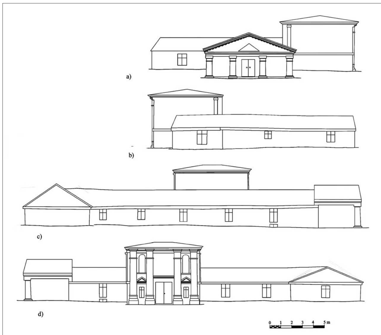
Рис. 134. Вірменський храм Аккермана. Фасади: а) західний; б) східний; в) північний; г) південний.
