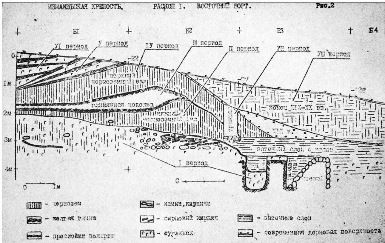
Рис. 97. Розріз валів Ізмайльської фортеці. Розкопки 1989 р. (Добролюбовский, Дынник 1990, с. 172-173).
