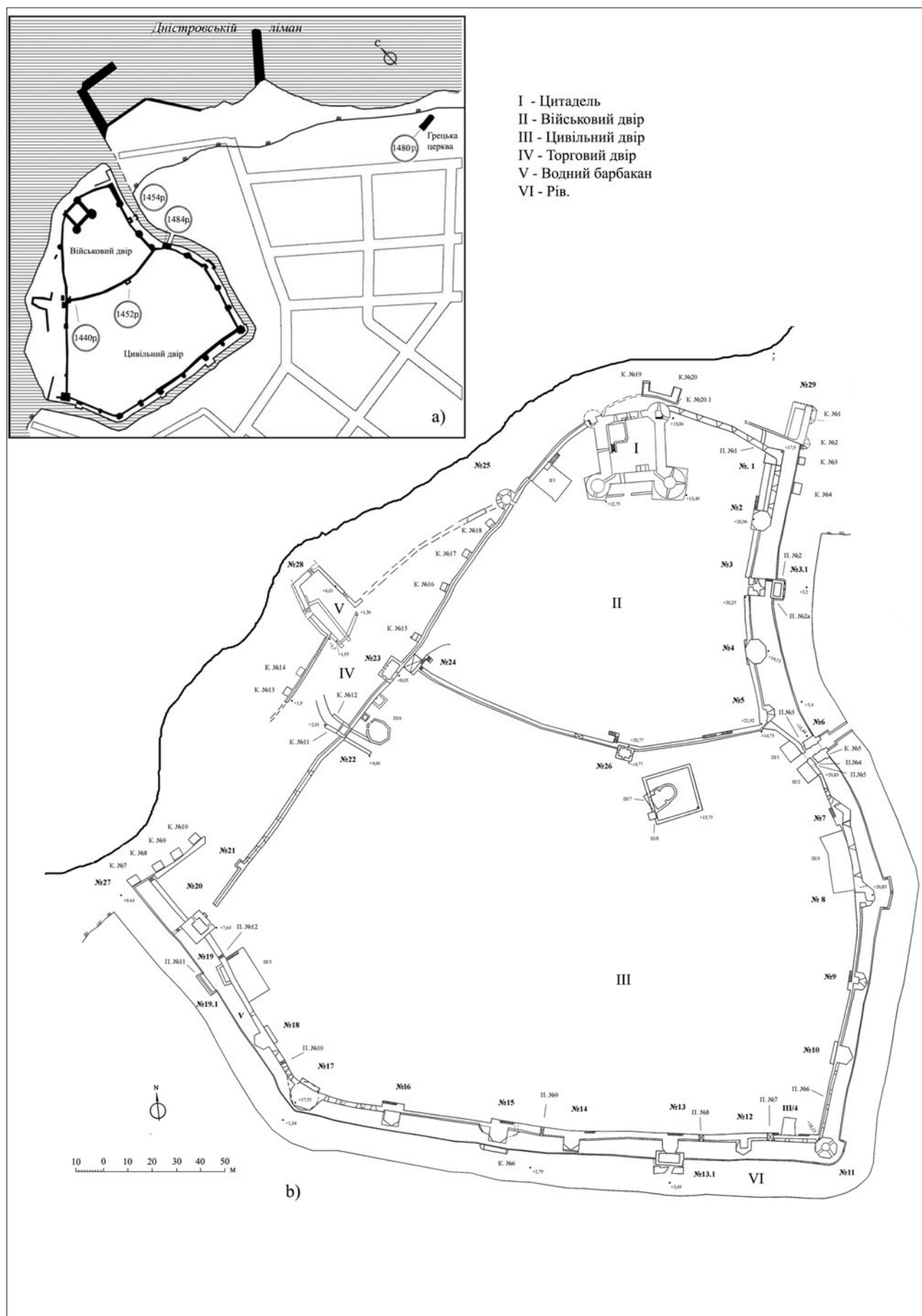
Рис. 18. Обмірний план фортеці Білгород (Аккерман) (б) з нумерацією веж та позначенням місць установки закладних плит (а).
