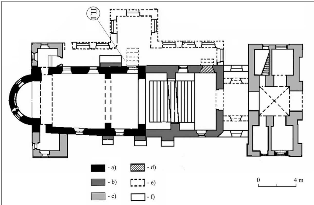
Рис. 154. Обмірний план церкви Св. Миколая (Nesterova 2010, p. 33).
