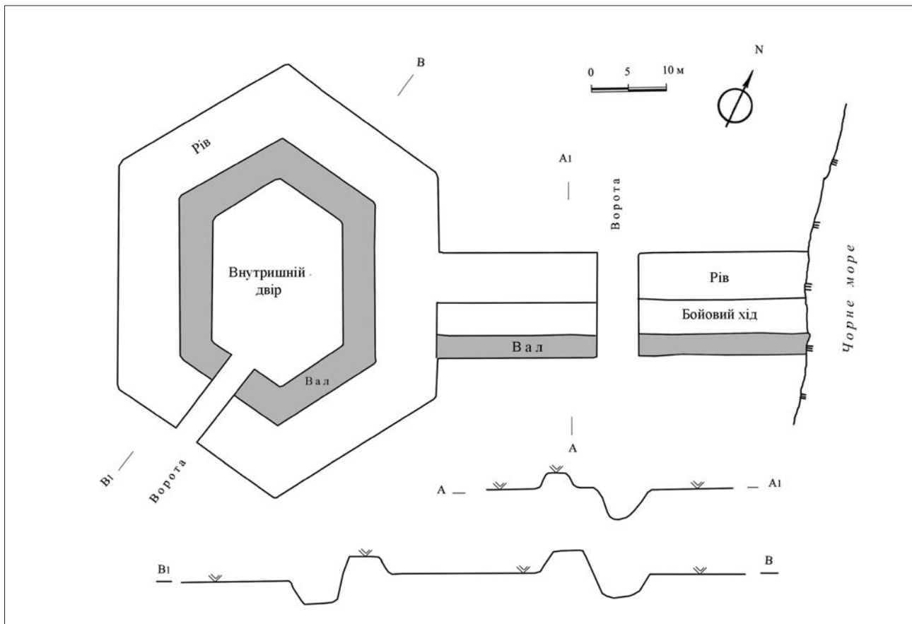
Рис. 122. Ситуаційний план Березанського форту.
