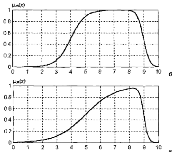
Рисунок 1.31 - Графіки П-подібних функцій приналежності \mu_{ПЗ}
